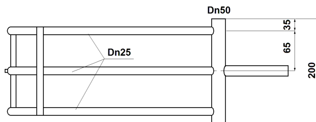
Wkład grzejny
